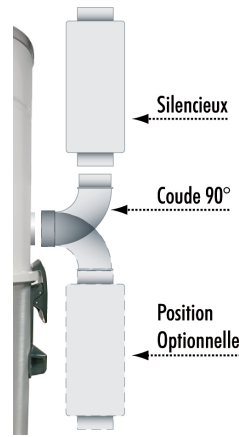
Fig.2 Installation du silencieux.
